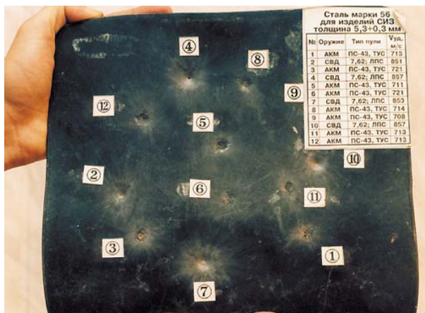
Стальная бронеплита после испытаний. По плите было сделано 12 выстрелов из автомата АКМ и снайперской винтовки Драгунова
