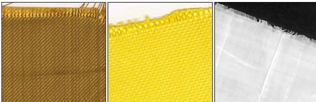
Образцы баллистических тканей, наиболее массово используемые в средствах индивидуальной бронезащиты (слева направо): «Кевлар» (TCBM), «Тварон», «Спектра»
