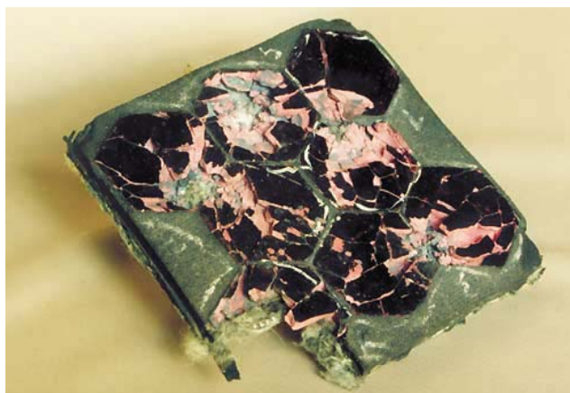
Керамический блок после испытаний. Блок выдержал 4 попадания, однако для него это предел. Все последующие попадания приведут к гарантированному пробитию
